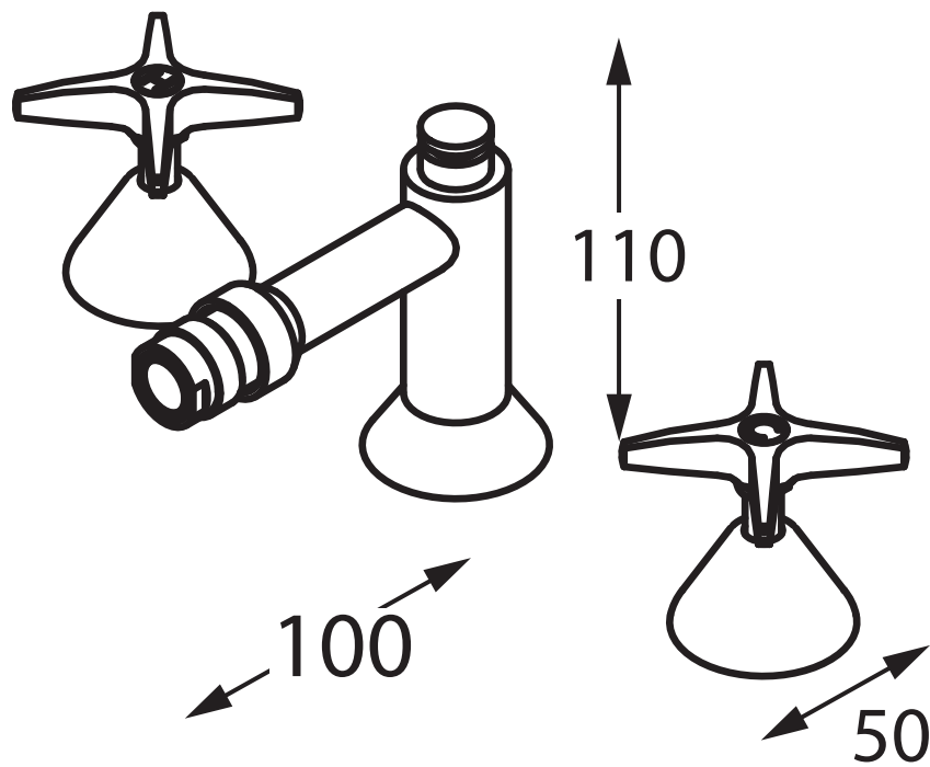
APP-C024 3/4N Bidette Set
